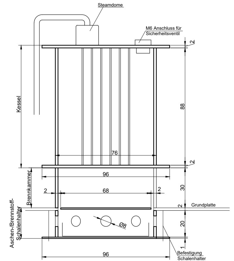
Schnitt
