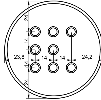
Querschnitt Kessel
