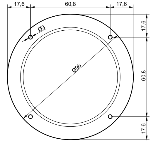
Bodenschalenhalter
