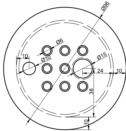
Abdeckplatte
